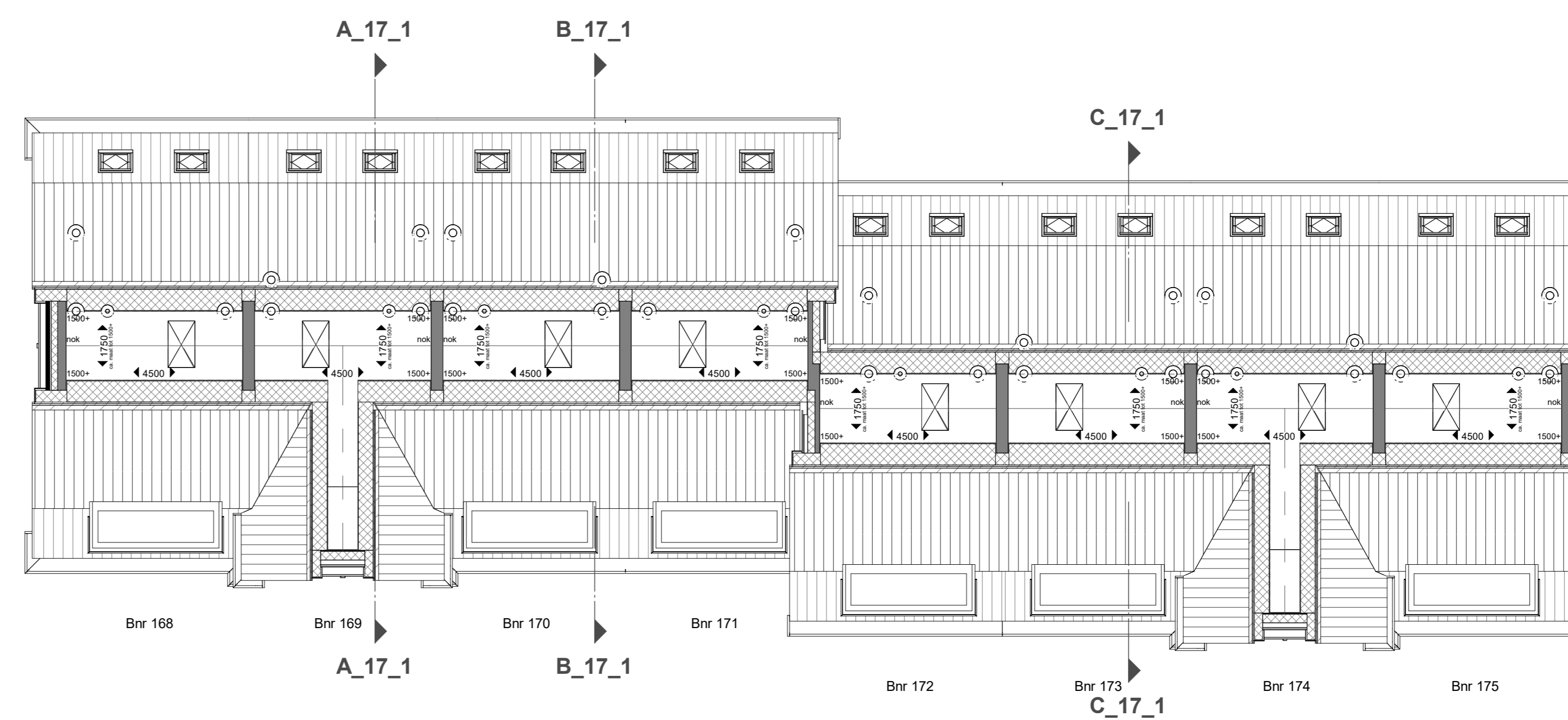
vliering
