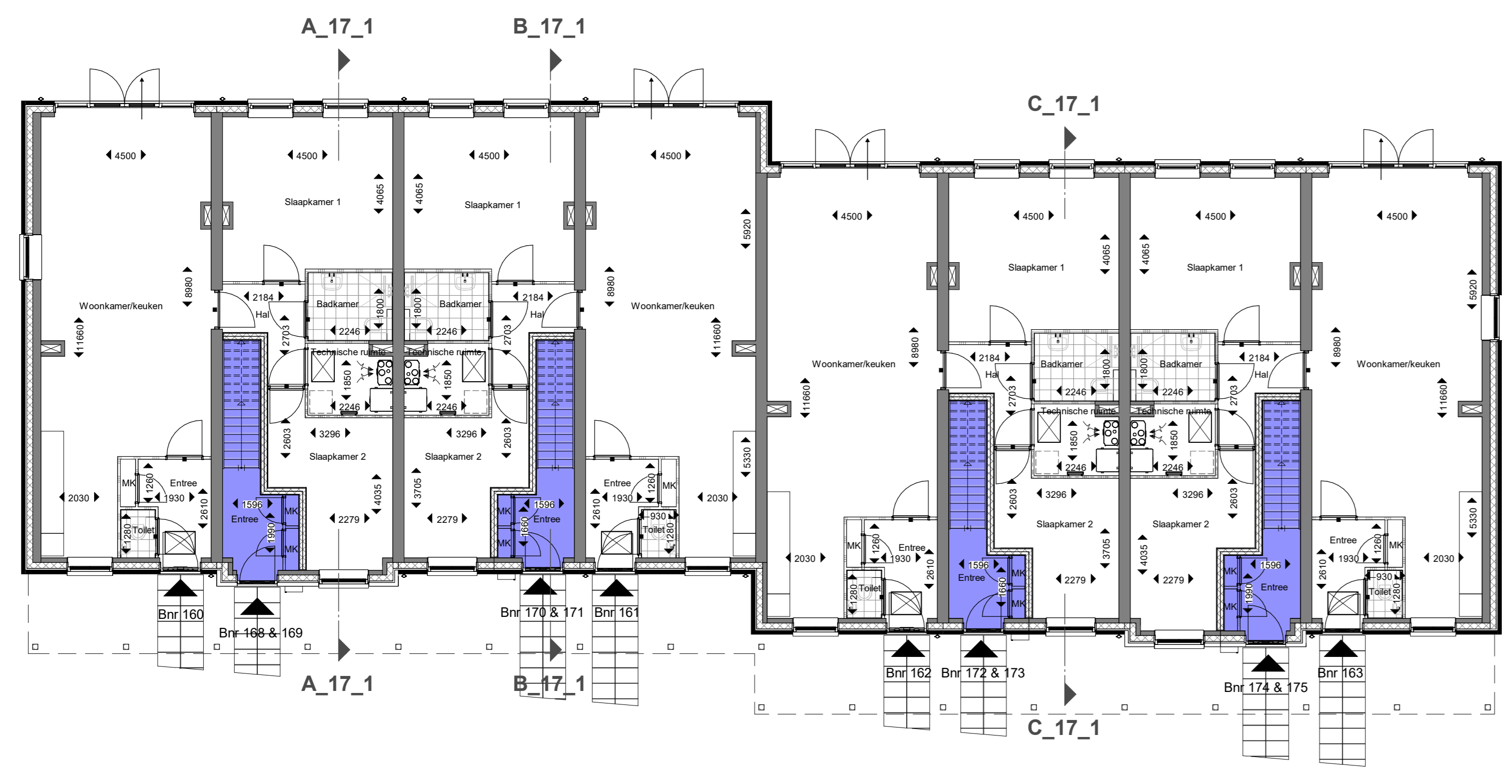
begane grond
